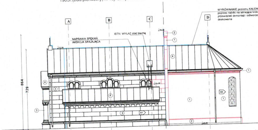
ELEVACJA Wschodnio - pn.
