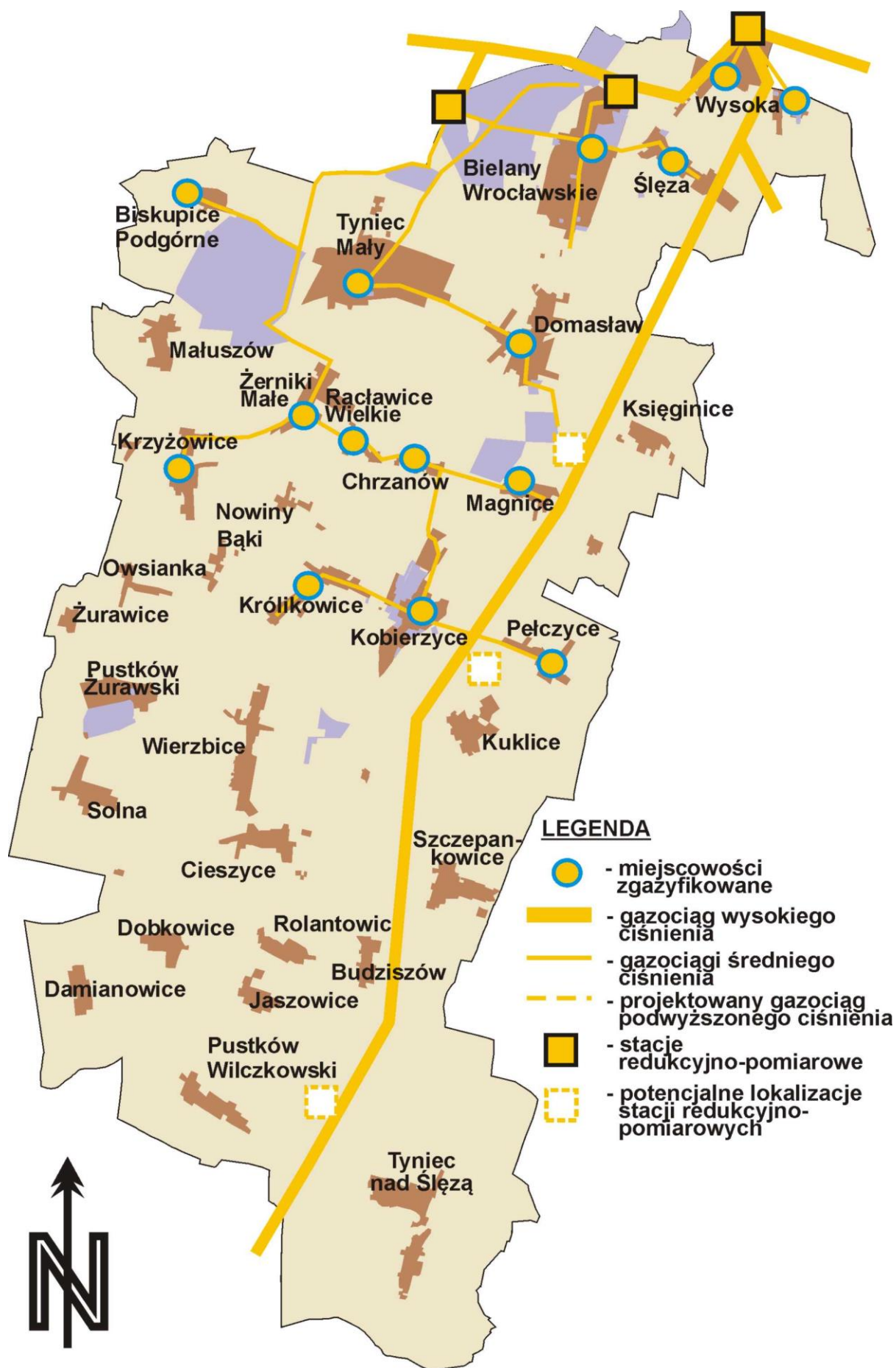
Rysunek 15 Sieć gazowa na terenie gminy Kobierzyce
