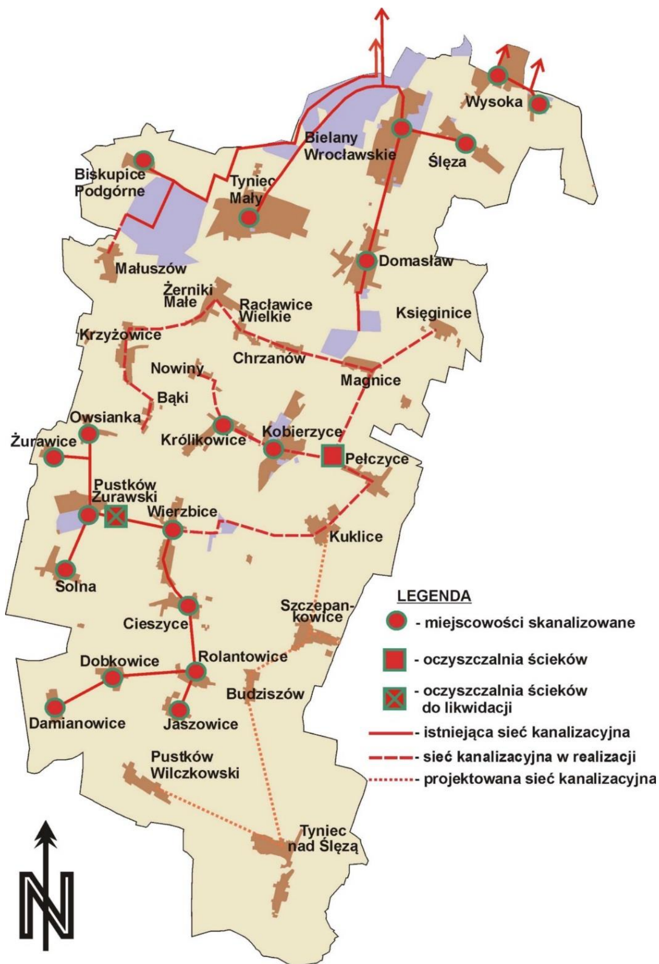
Rysunek 14 Sieć kanalizacyjna w gminie Kobierzyce
